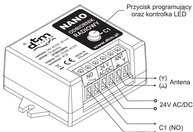
Rys. 1. Widok odbiornika radiowego z opisem połączeń.
